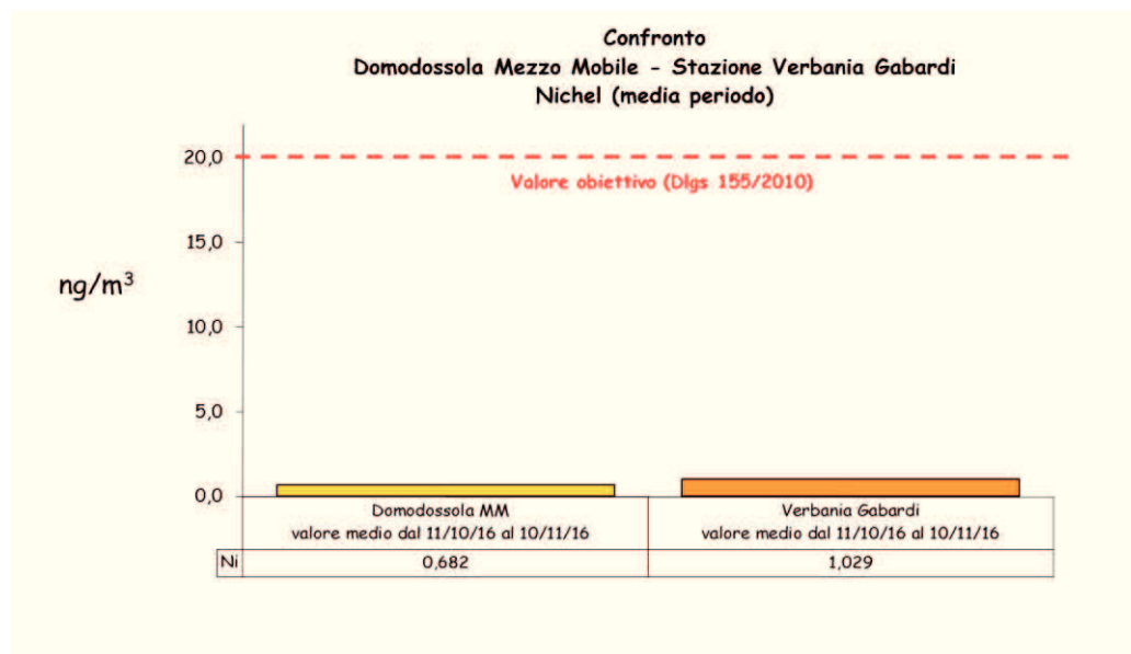
Figura 35: confronto tra Domodossola Mezzo Mobile e Stazione di Verbania Gabardi
