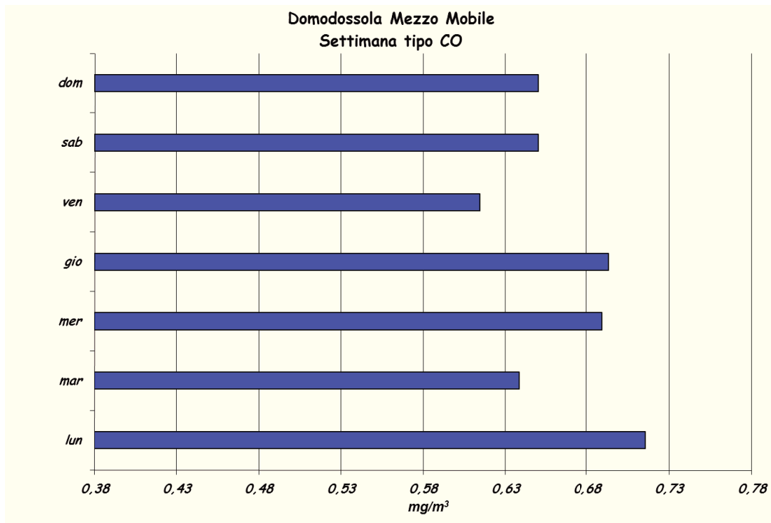
Figura 14: Monossido di Carbonio - settimana tipo
