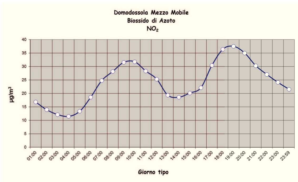
Figura 18: Biossido di azoto - giorno tipo
