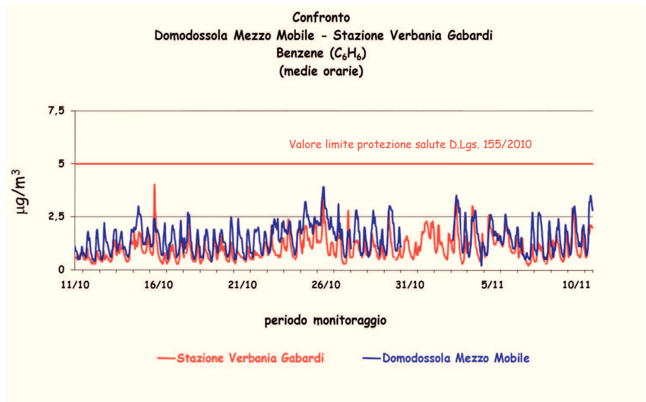
Figura 24: valori orari Benzene
