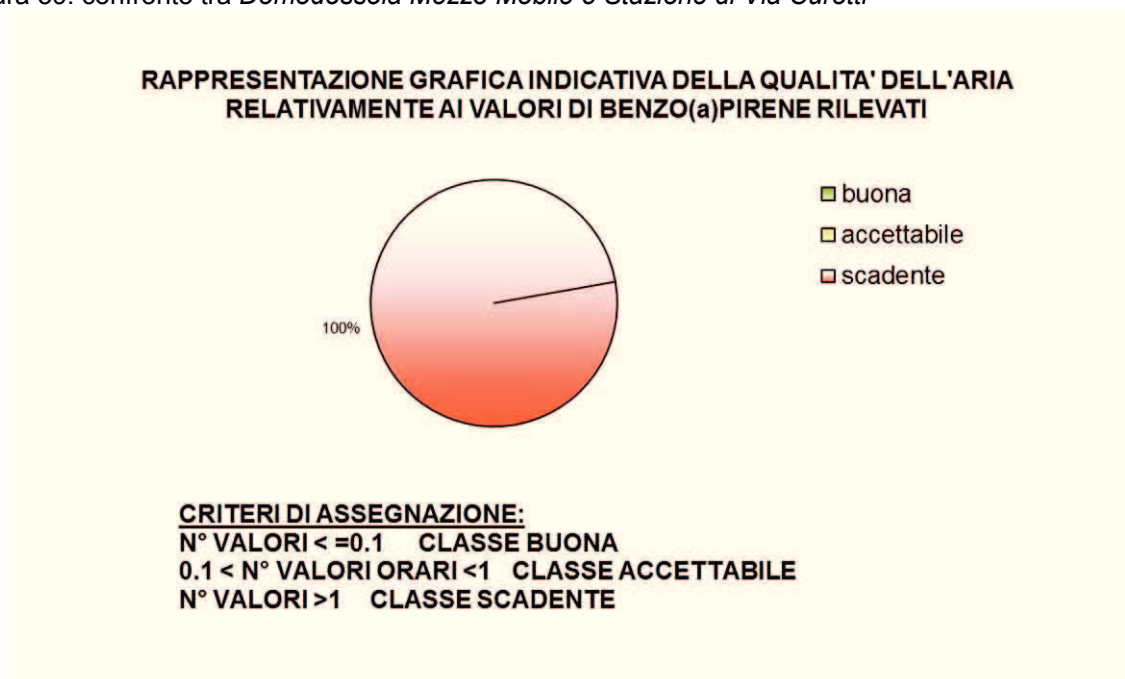
Figura 40: giudizio sulla qualità dell'aria relativo a Benzo(a)pirene.
