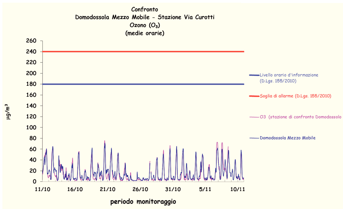
Figura 20: medie orarie Ozono
