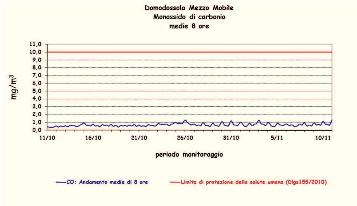
Figura 12: medie mobile otto ore di Monossido di Carbonio
