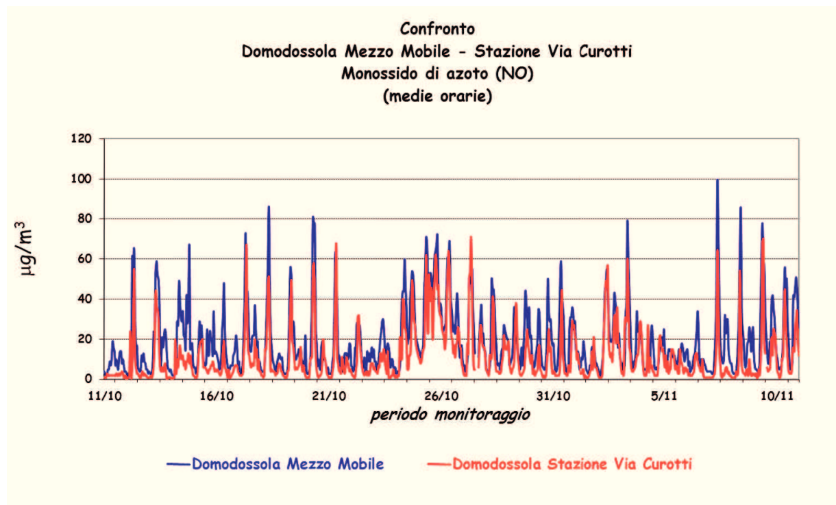
Figura 23: medie orarie Monossido di Azoto
