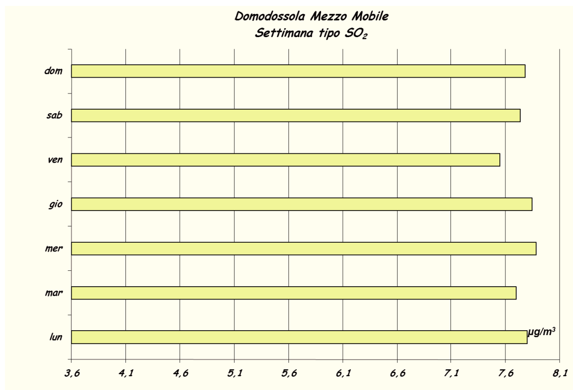
Figura 9: settimana tipo Biossido di Zolfo
