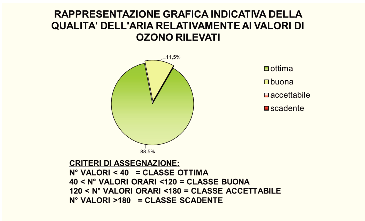
Figura 22: giudizio sulla qualità dell'aria relativo ad Ozono
