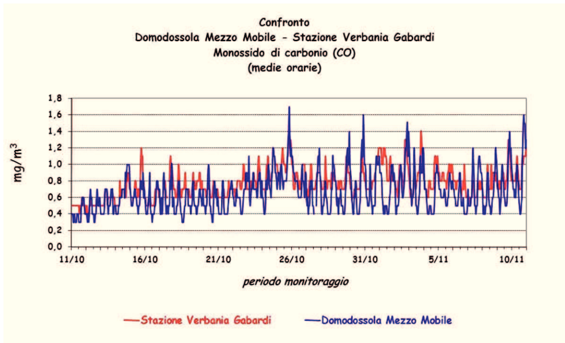
Figura 11: medie orarie Monossido di Carbonio
