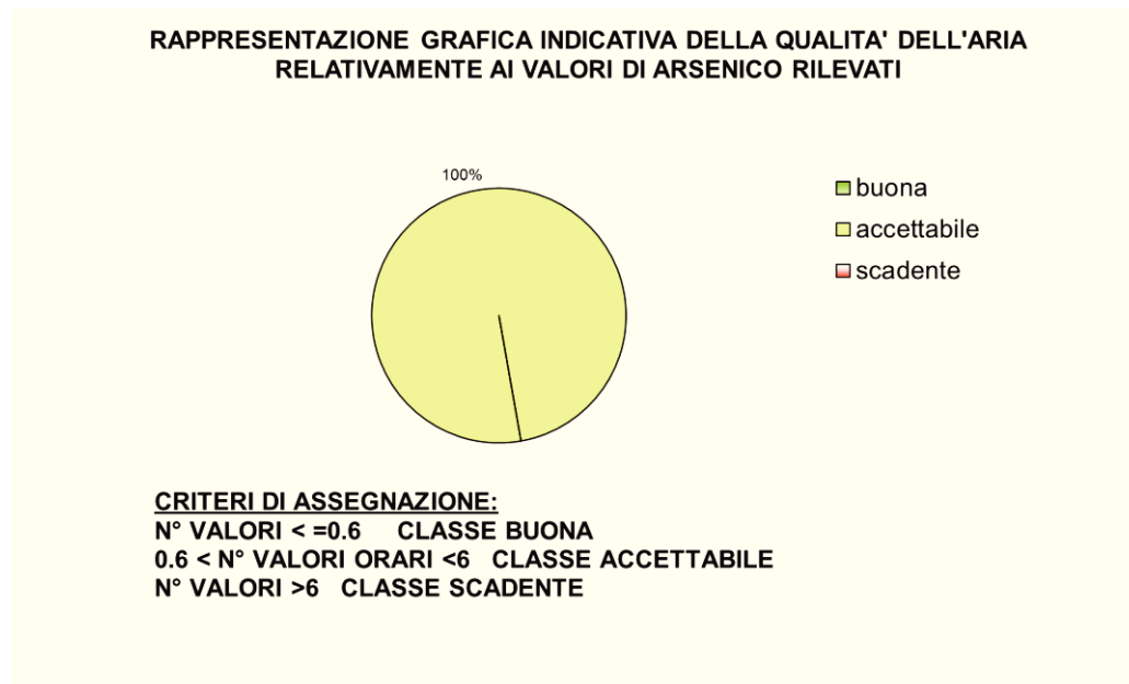
Figura 32: giudizio sulla qualità dell'aria relativo ad Arsenico
