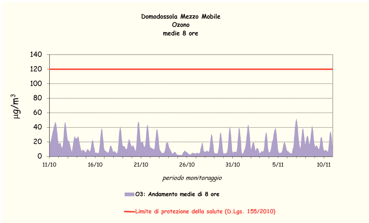
Figura 21: medie mobili otto ore Ozono
