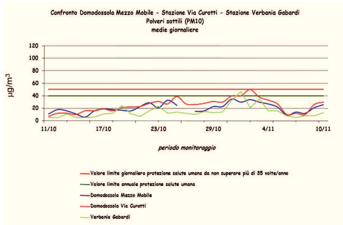
Figura 28: valori giornalieri di PM10
