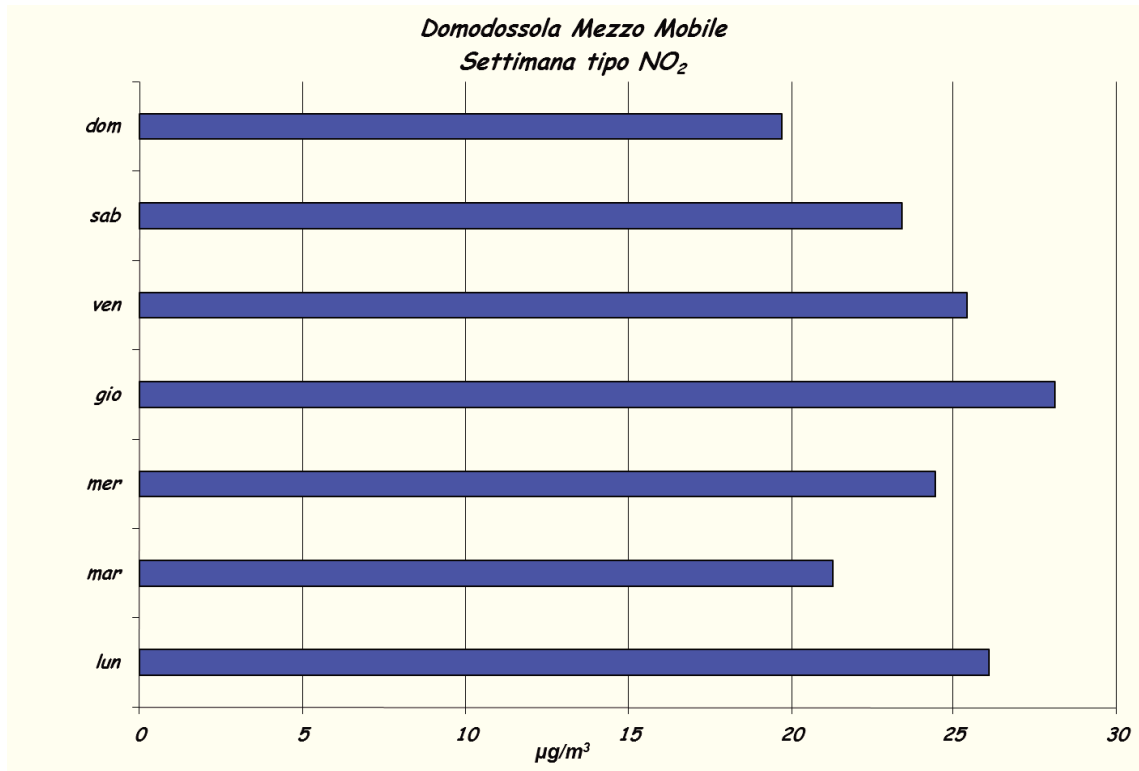
Figura 17: variabilità settimanale media giornaliera di NO 2
