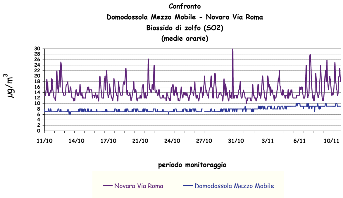
Figura 8: medie orarie Biossido di Zolfo
