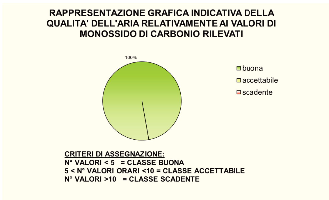
Figura 15: giudizio sulla qualità dell'aria relativo al Monossido di Carbonio
