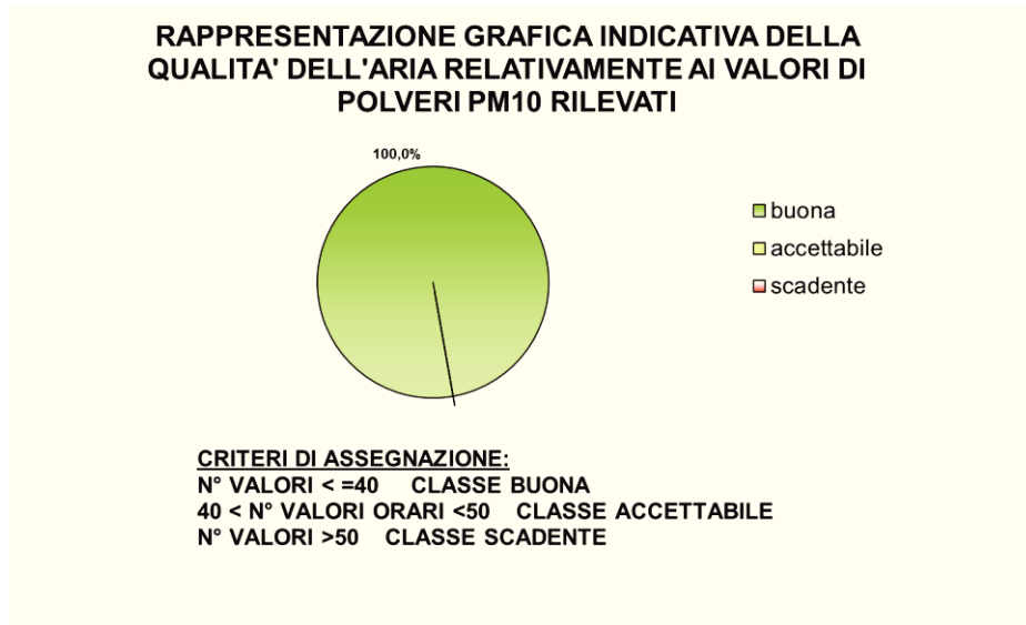
Figura 29: giudizio sulla qualità dell'aria relativo ai valori giornalieri di PM10
