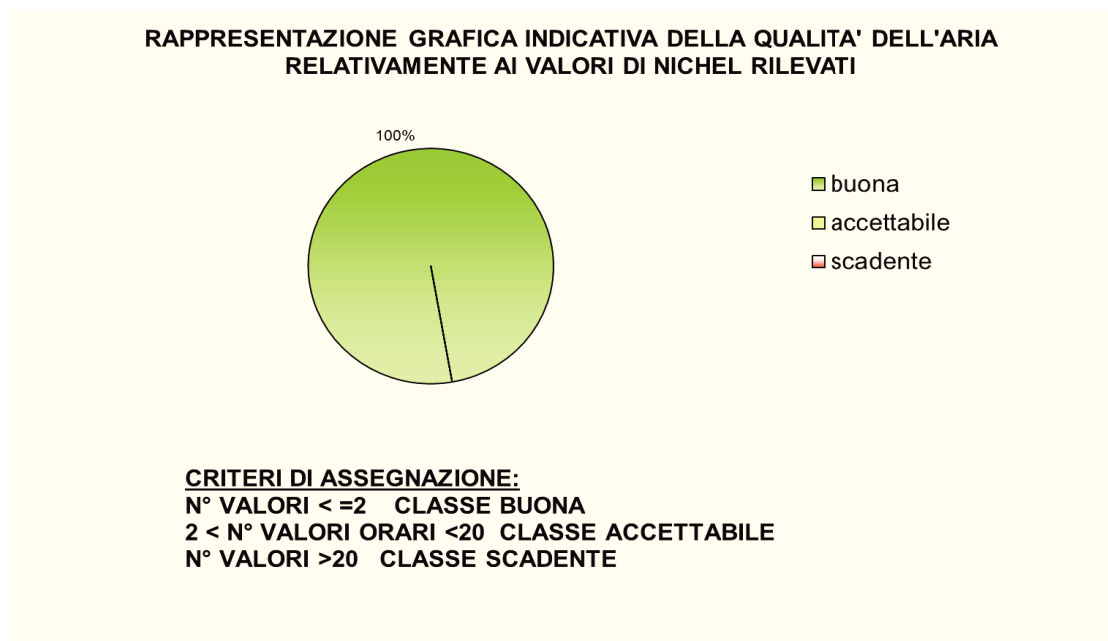
Figura 36: giudizio sulla qualità dell'aria relativo al Nichel.
