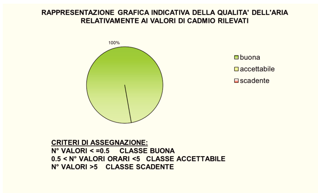
Figura 34: giudizio sulla qualità dell'aria relativo al Cadmio.
