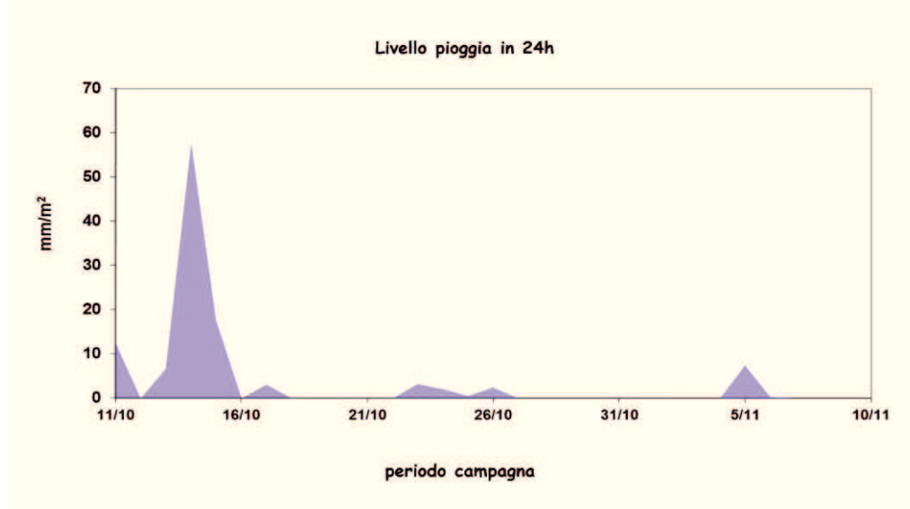
Figura 42: valori giornalieri di pioggia caduta.
