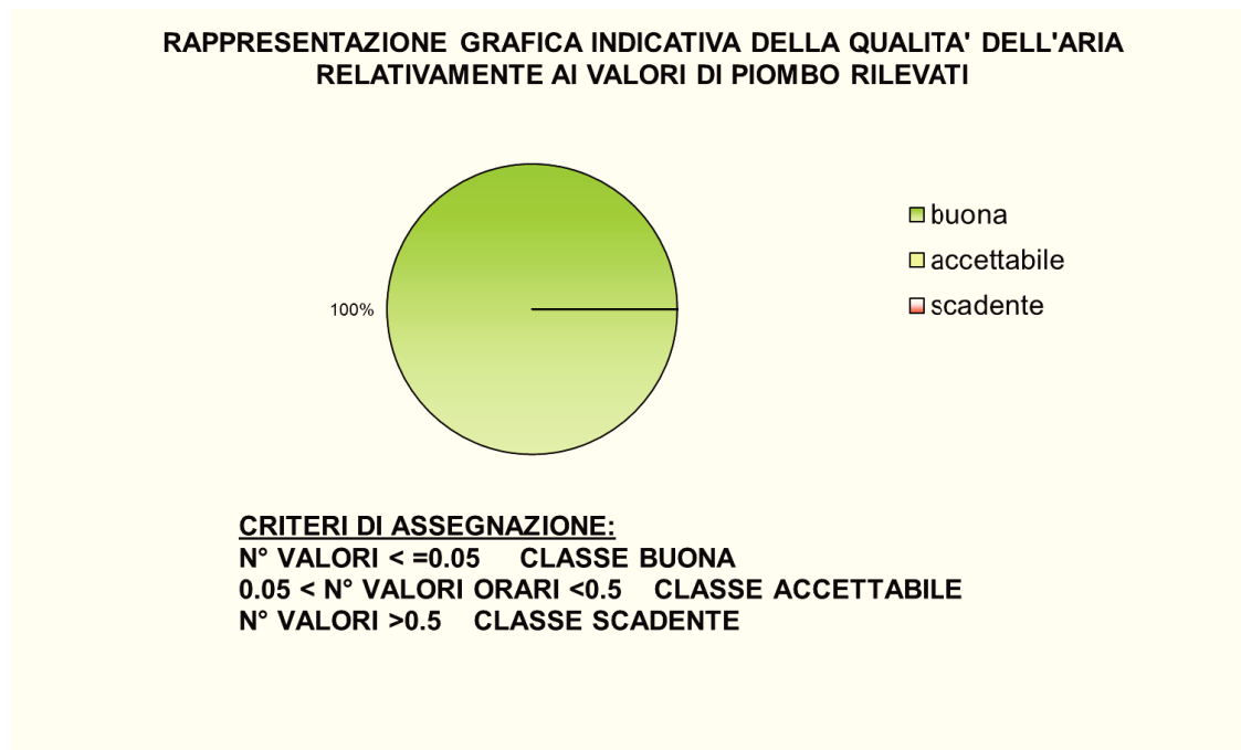
Figura 38: giudizio sulla qualità dell'aria relativo al Piombo.
