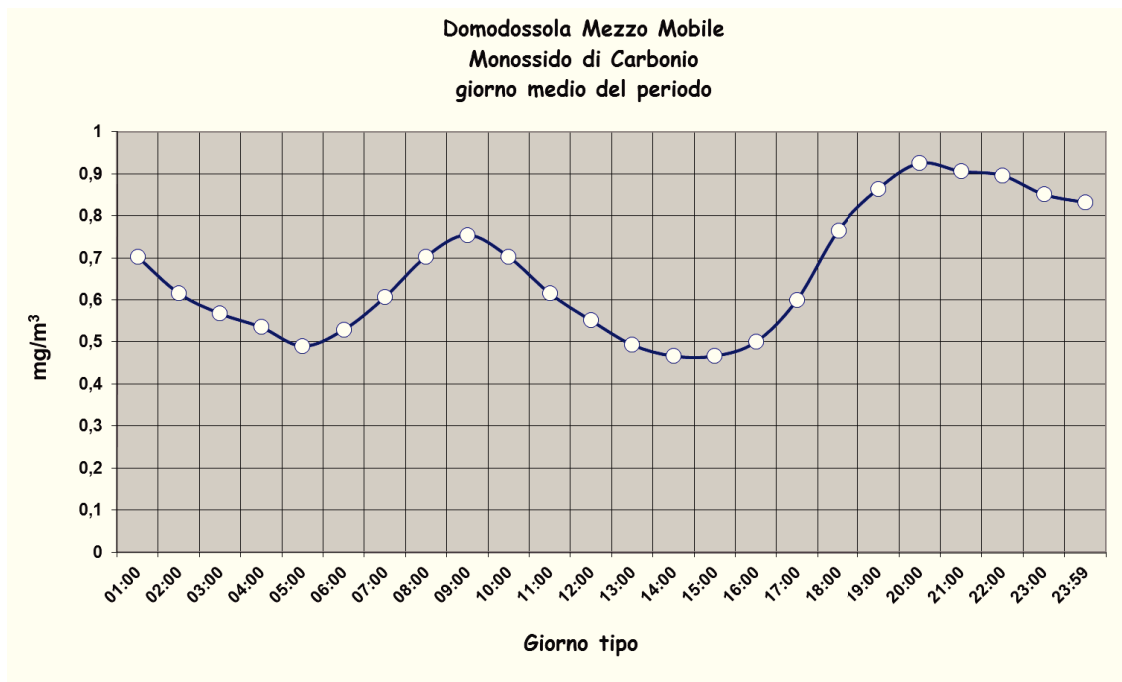
Figura 13: Monossido di Carbonio - giorno tipo
