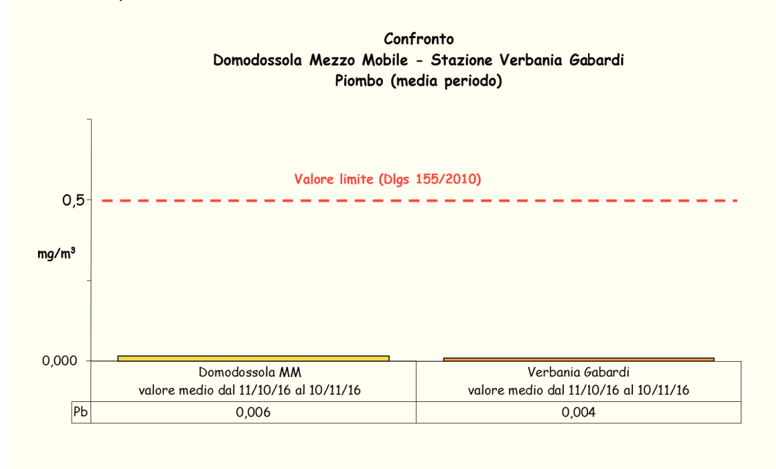
Figura 37: confronto tra Domodossola Mezzo Mobile e Stazione di Verbania Gabardi
