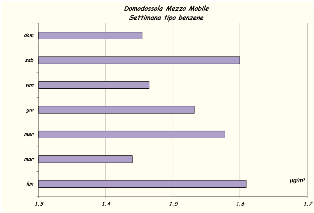
Figura 26: Benzene - settimana tipo
