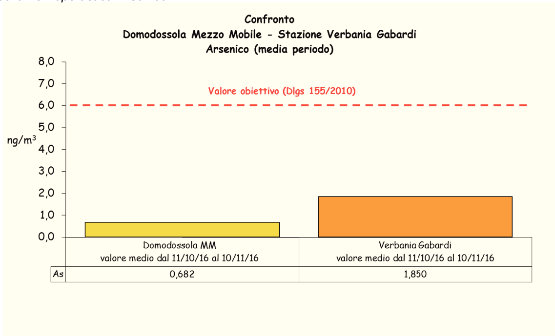
Figura 31: confronto tra Domodossola Mezzo Mobile e Stazione di Verbania Gabardi
