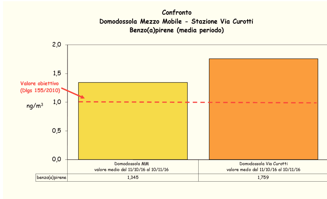
Figura 39: confronto tra Domodossola Mezzo Mobile e Stazione di Via Curotti
