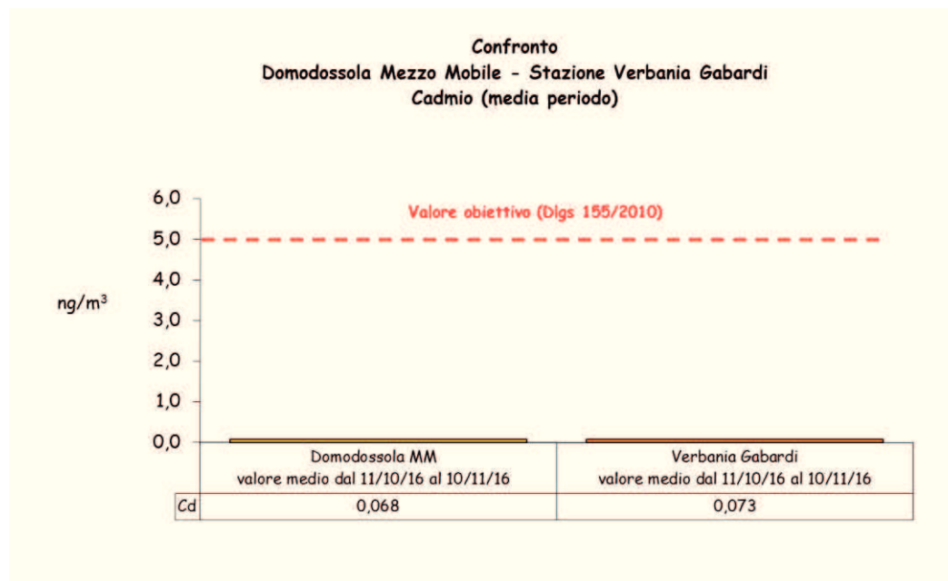
Figura 33: confronto tra Domodossola Mezzo Mobile e Stazione di Verbania Gabardi
