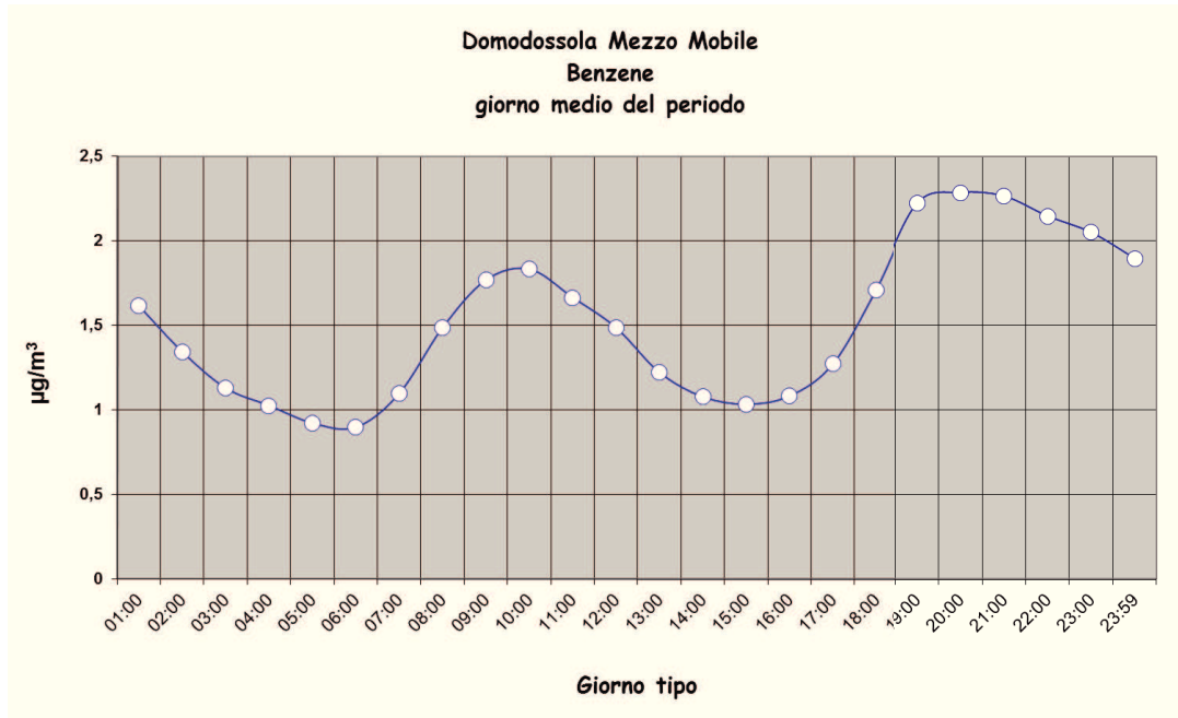
Figura 25: Benzene – giorno tipo
